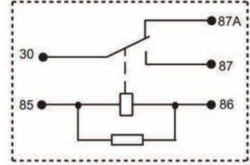
JTV4H/□□□-1Z□□□R(XXX)
