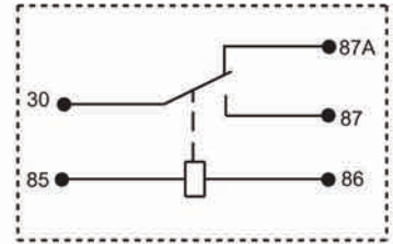
JTV4H/□□□-1Z□□□(XXX)
