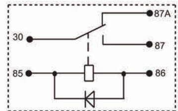
JTV4H/□□□-1Z□□□D1(XXX)
