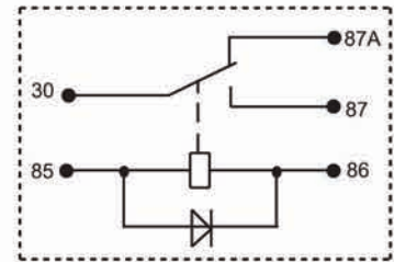
JTV4H/□□□-1Z□□□D2(XXX)
