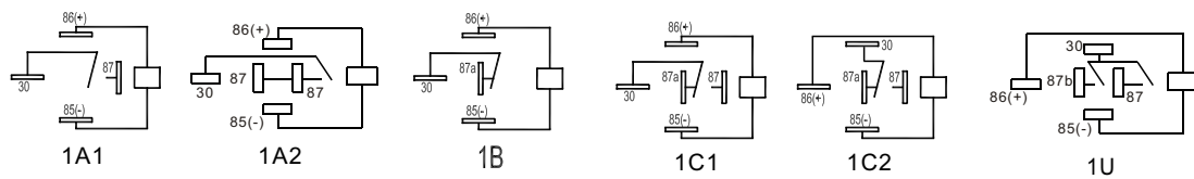
接线图 (底视图)
