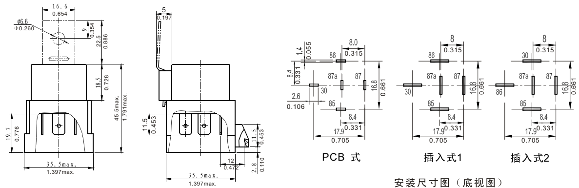
安装尺寸图 (底视图)
