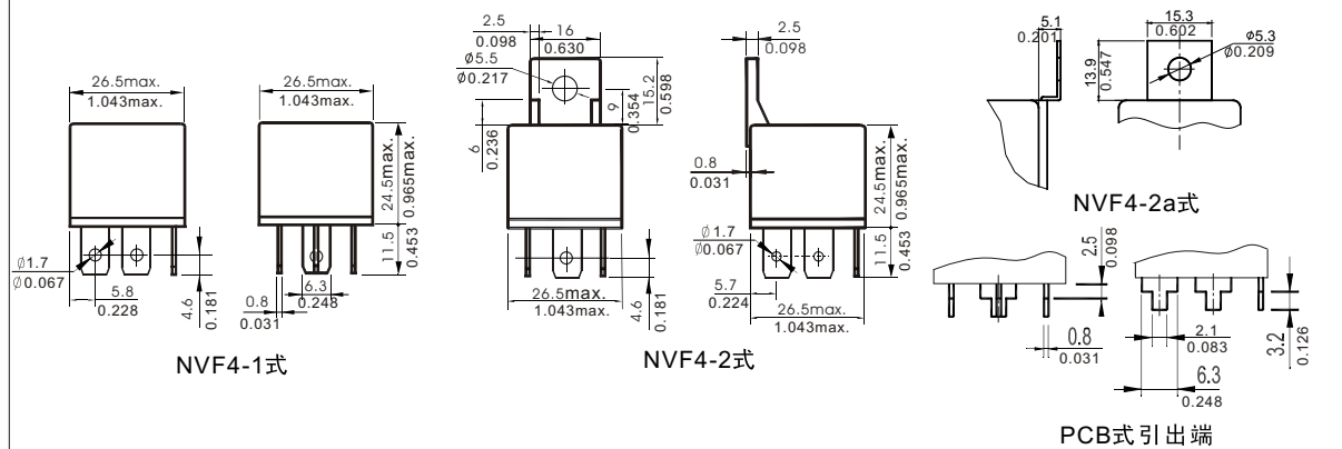
外形尺寸图
