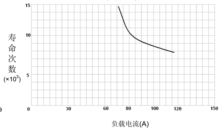
寿命曲线
