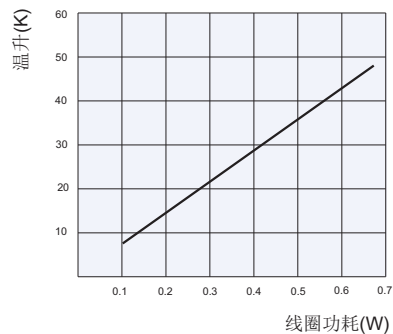
线圈温升
