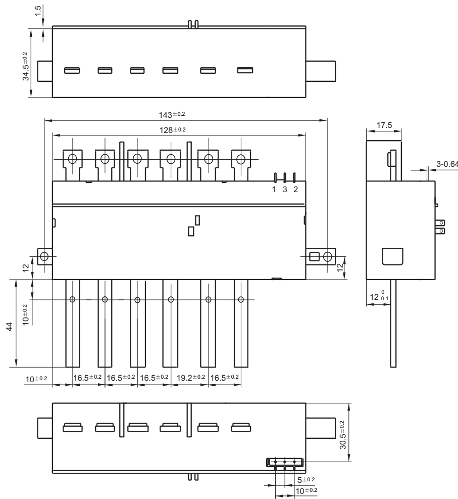
外形图
