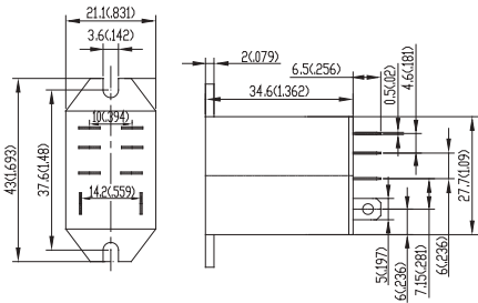
Flange Top Type 法兰式 Socket Terminal 插座式端子
