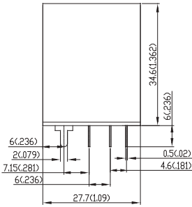
Flange Top Type 法兰式 Socket Terminal 插座式端子
